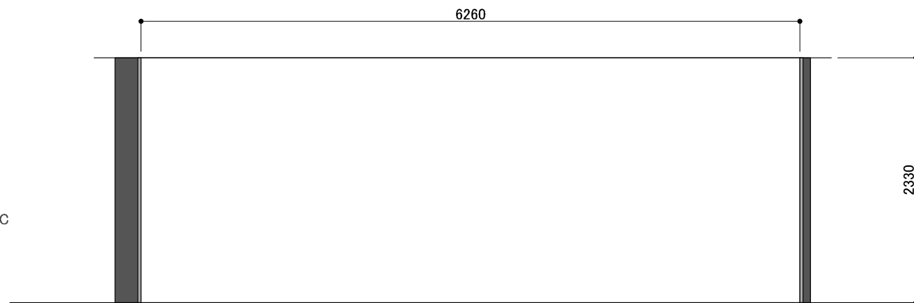
A-A展開
