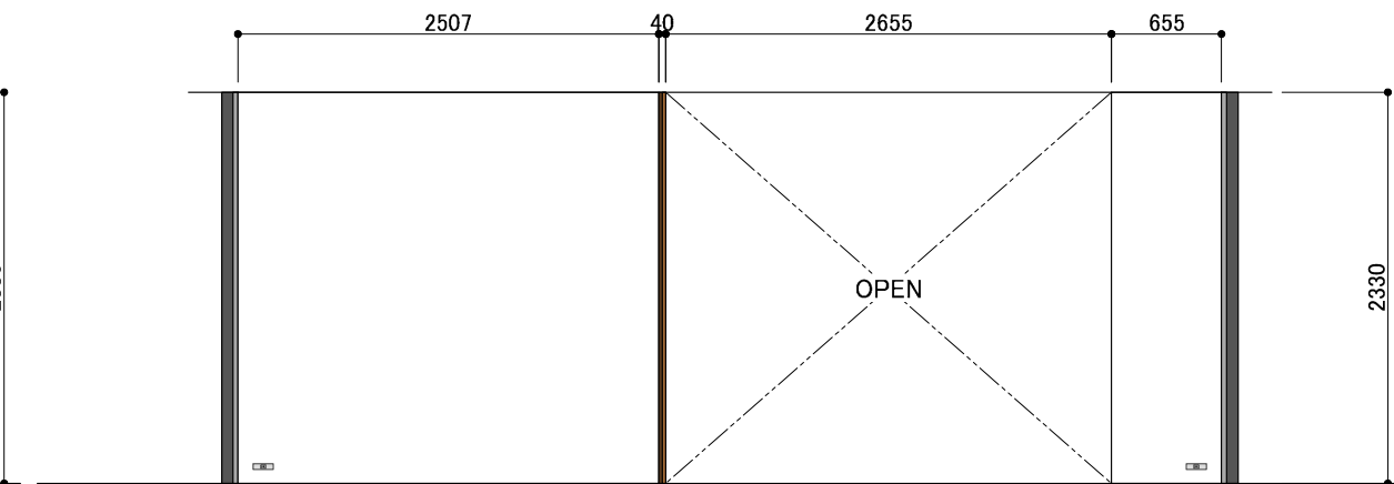
B-B展開
